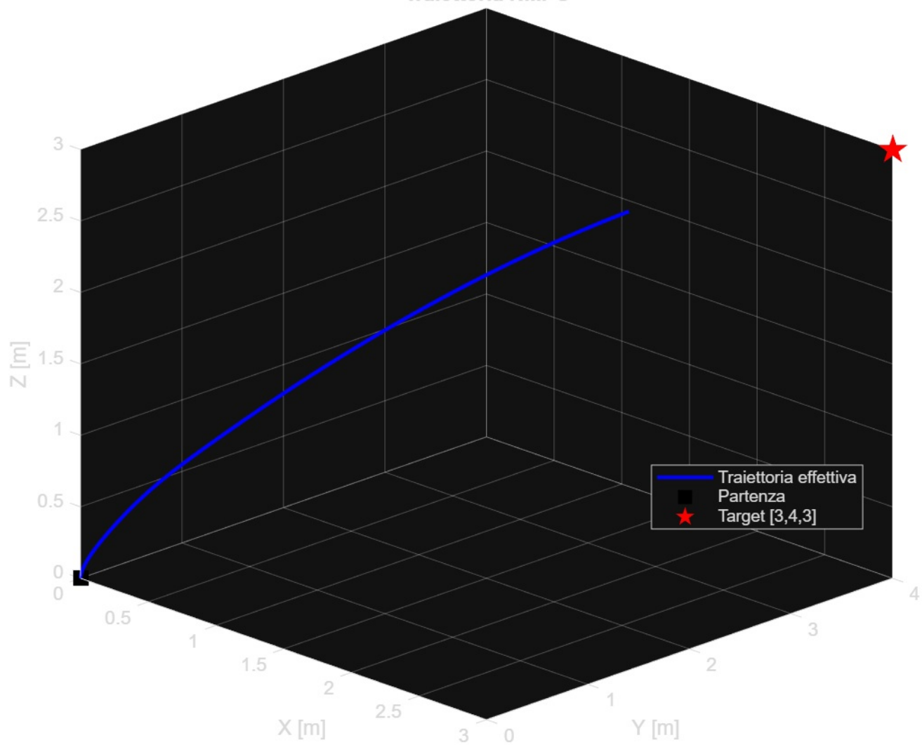
Traiettoria NMPC
